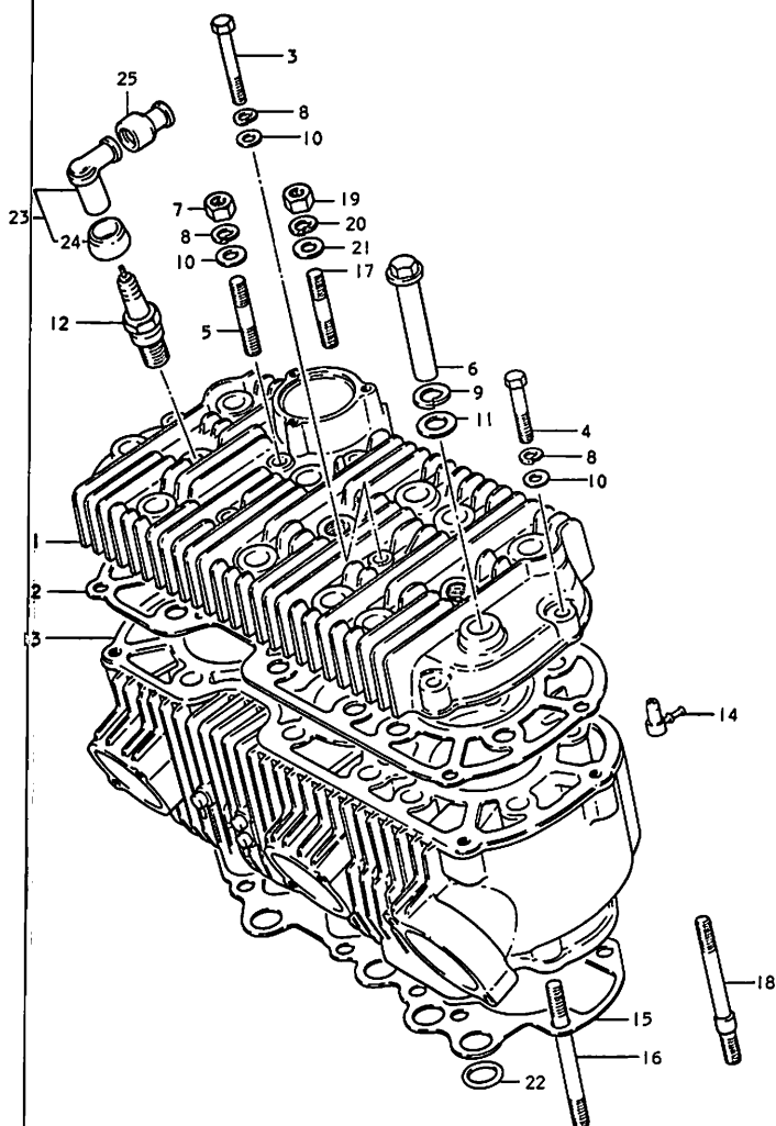
FIG. 3 シリンダ (B4, B5)
