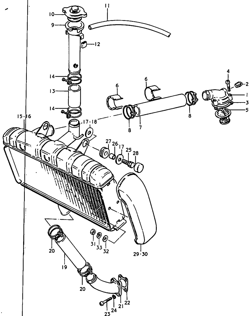
FIG. 20 ラジエータ
