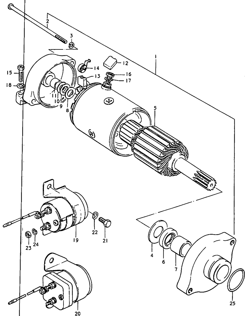
FIG. 26 スターティング モータ (日本電装製)
