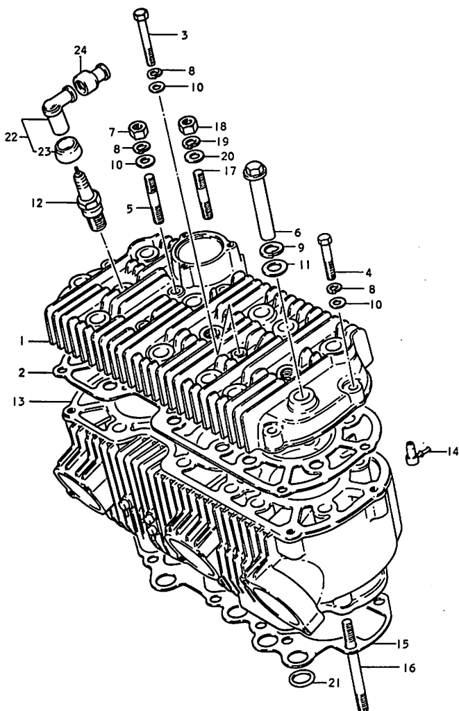
FIG. 1 シリンダ (GT750)
