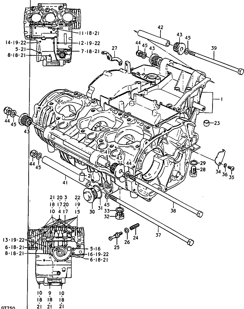
FIG. 4 クランクケース
