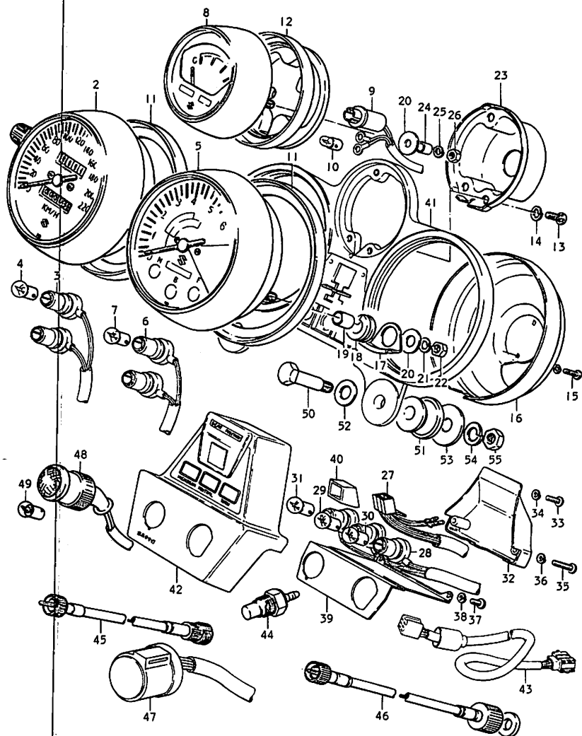
FIG. 31 コンビネーションメータ (B3,B4,B5)
