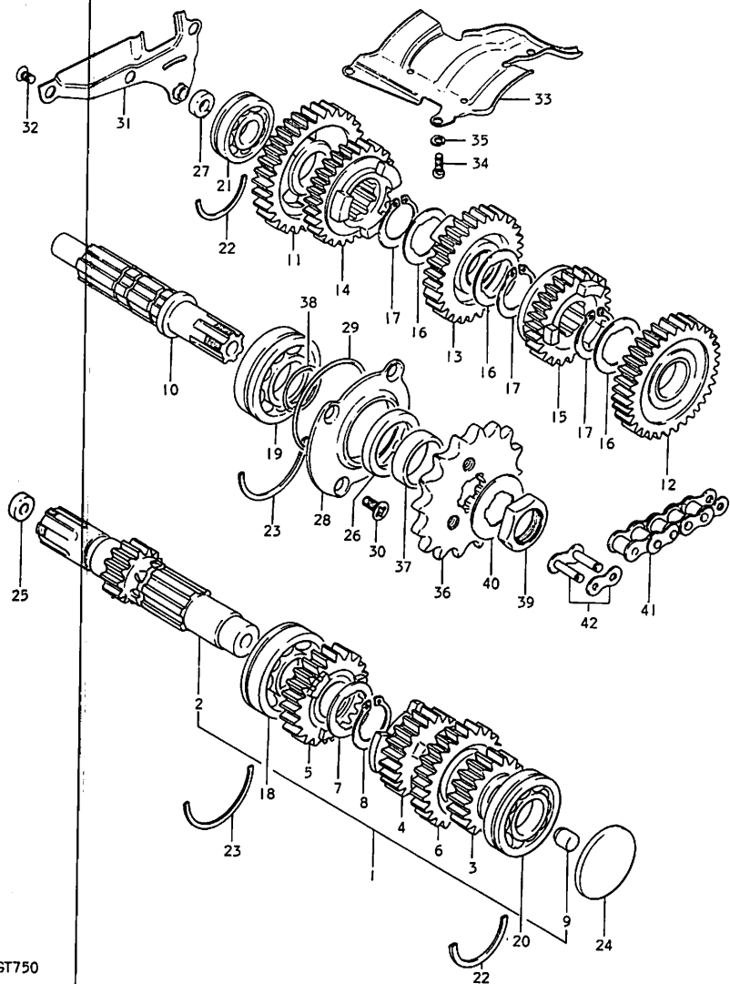
FIG. 23 トランスミッション
