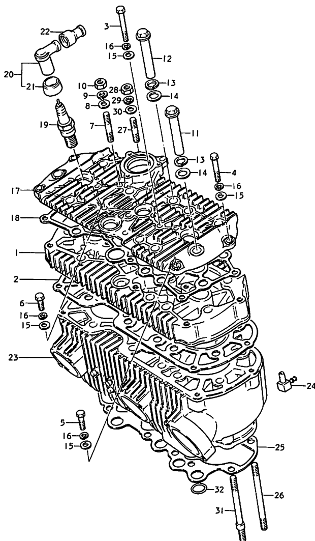
FIG. 2 シリンダ (B1,B3)
