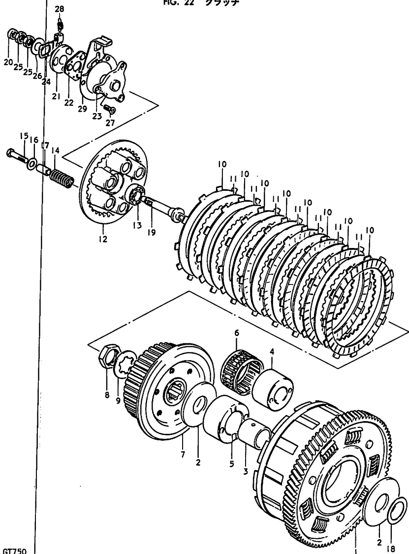
FIG. 22 クラッチ
