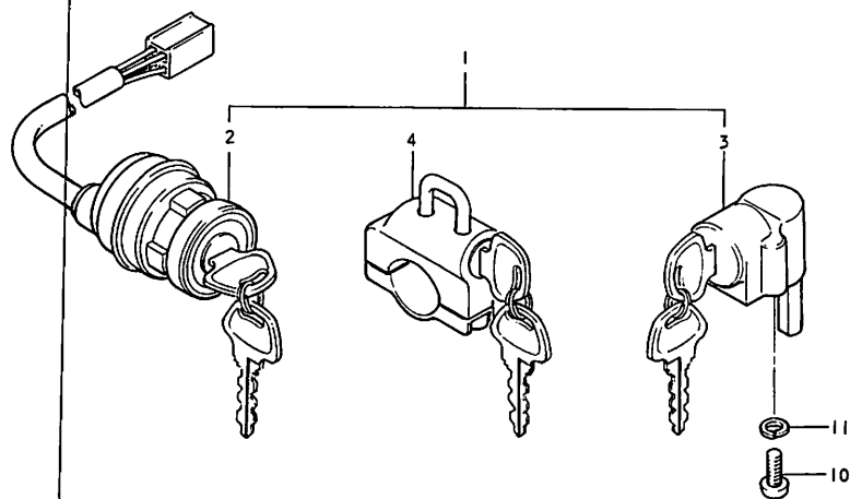
FIG. 41 ロック セット
