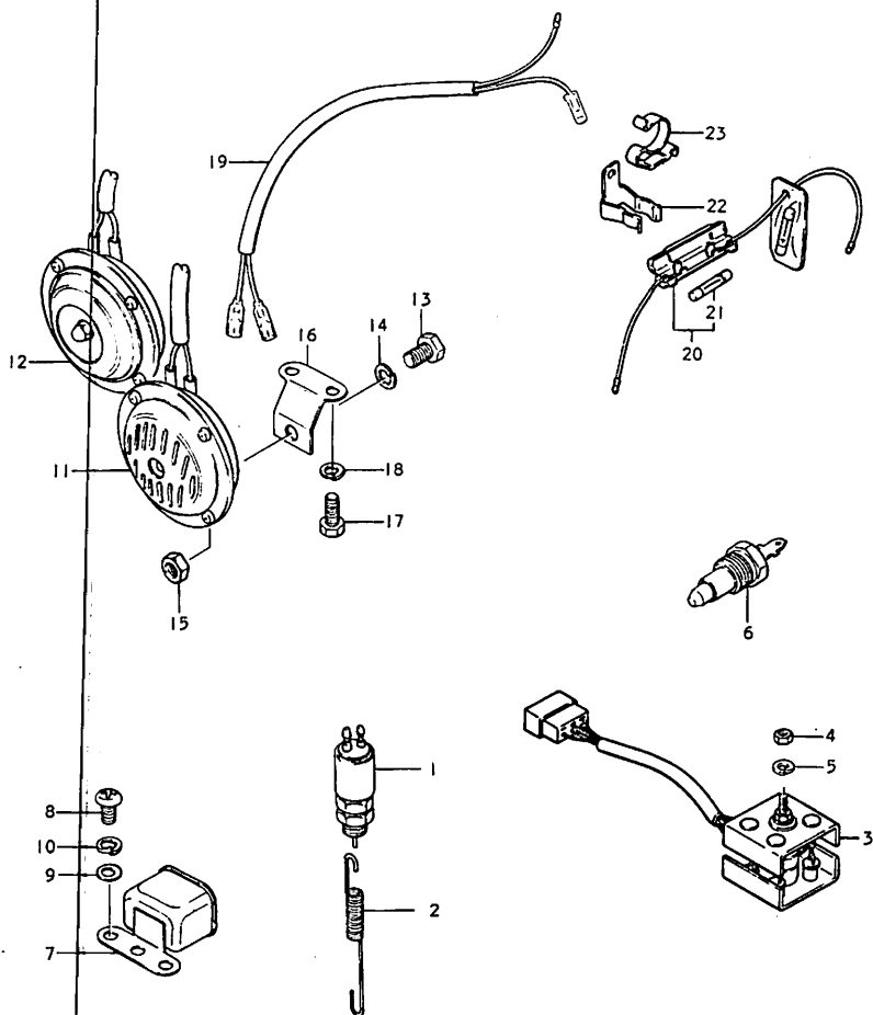
FIG. 40 エレクトリカル
