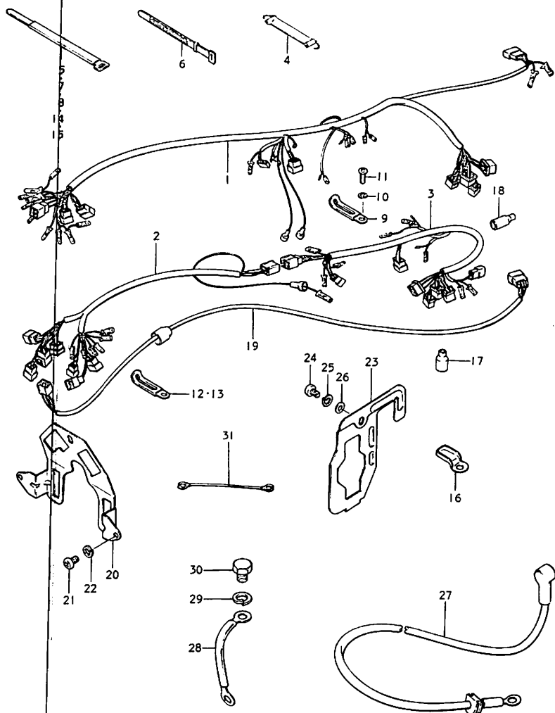
FIG. 38 ワイヤリング ハーネス
