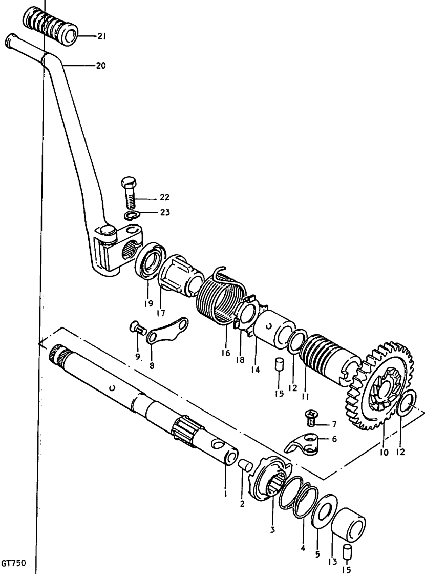
FIG. 25 キック スタータ
