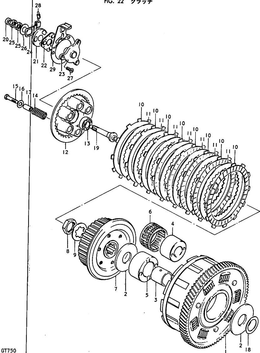
FIG. 22 クラッチ
