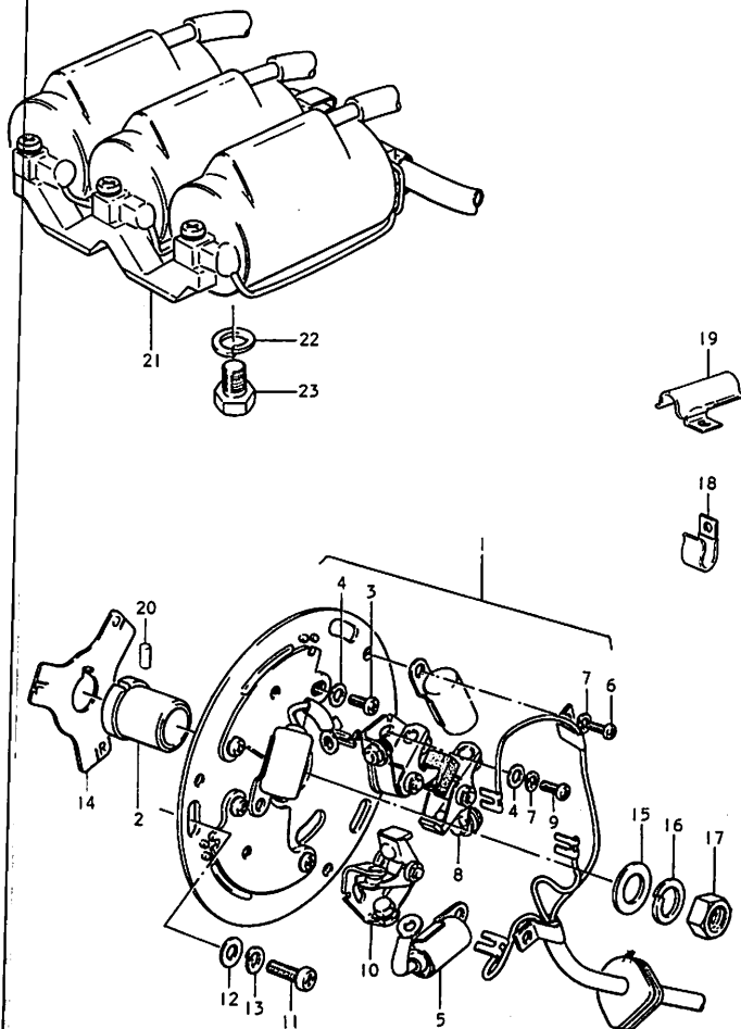
FIG. 29 コンタクト ブレーカ
