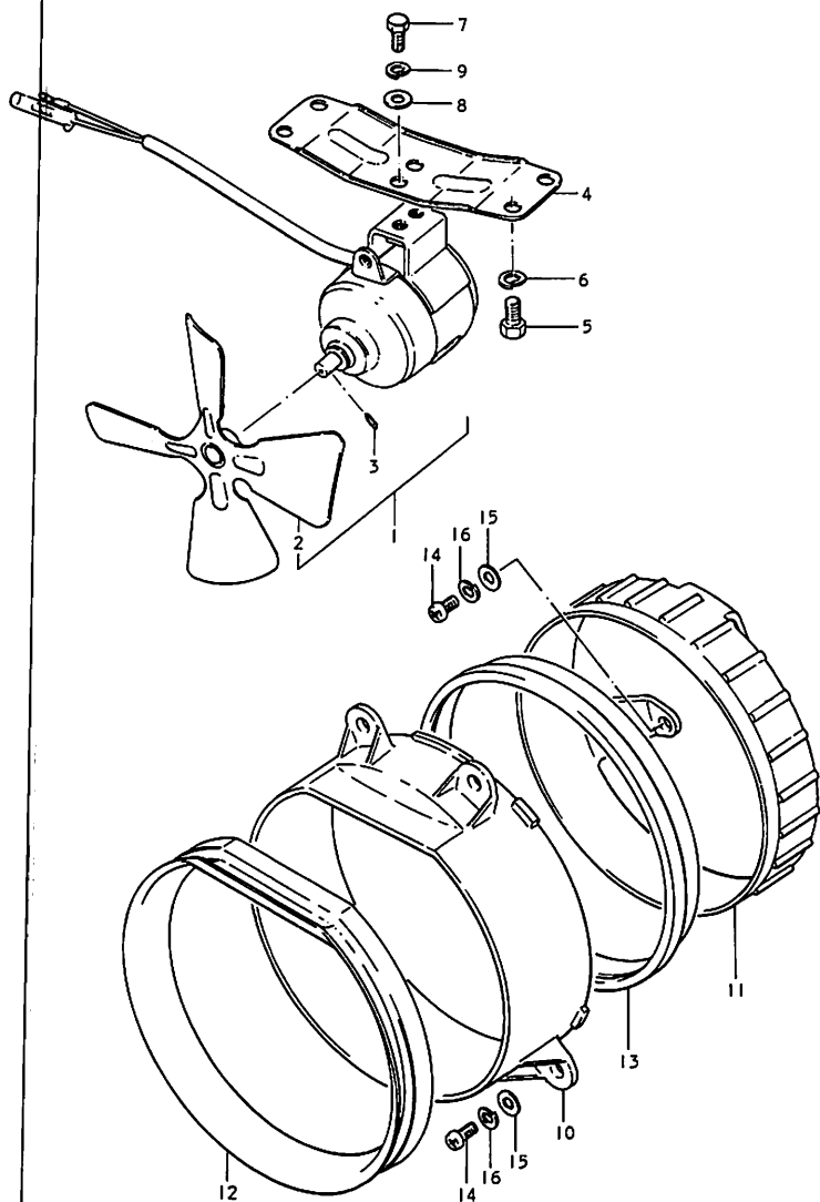
FIG. 18 クーリング ファン
