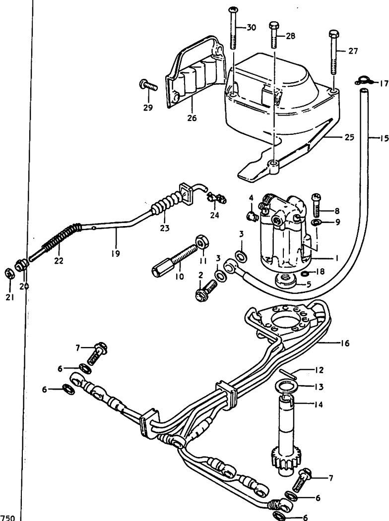
FIG. 15 オイル ポンプ
