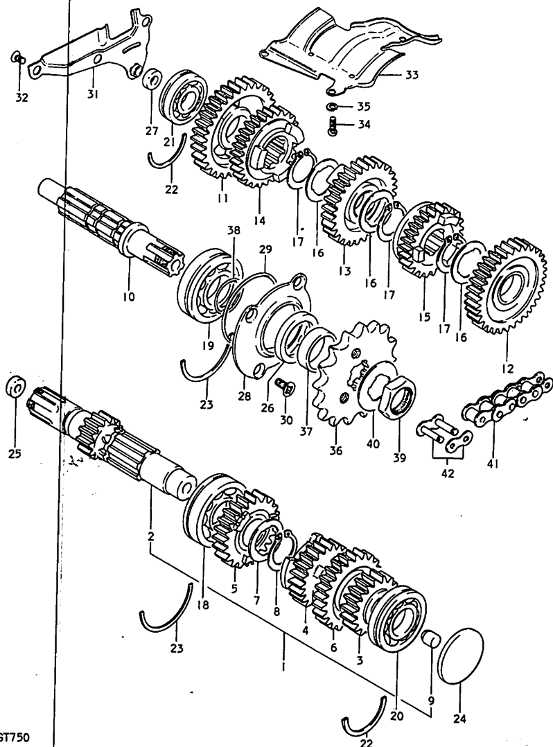
FIG. 23 トランスミッション
