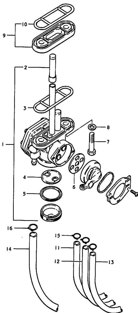
FIG. 51 フューエル コック
